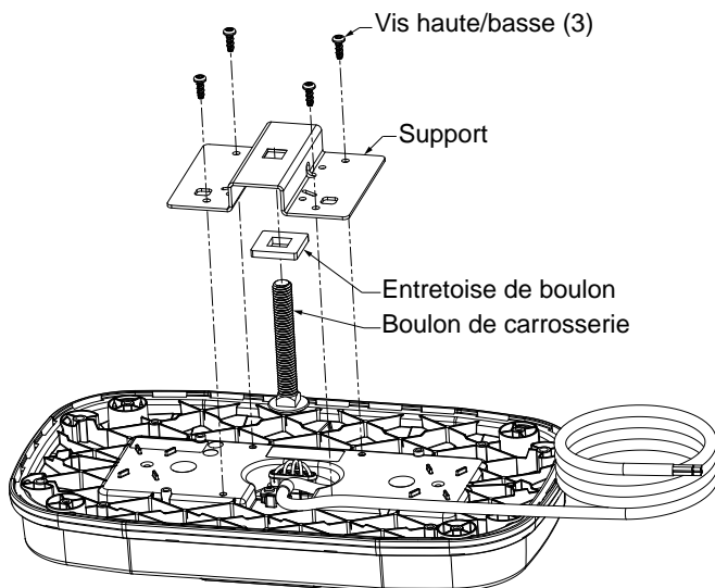
Figure 5 : Fixation du support de montage de feux d'aile HighLighter Elite
